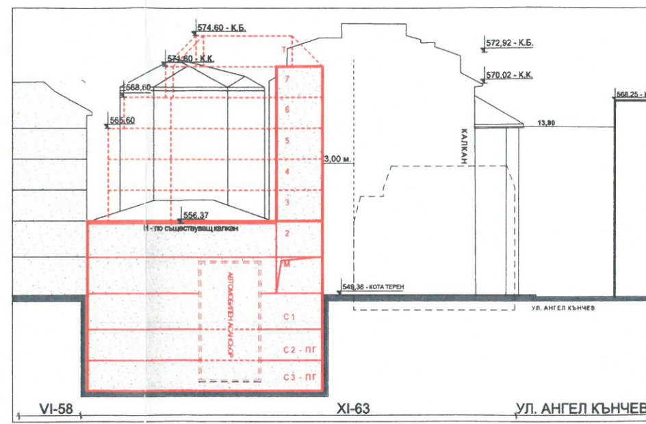
РАЗРЕЗ 2-2 М 1:500
