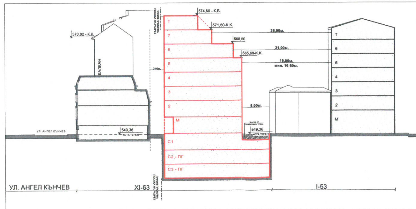
РАЗРЕЗ 1-1 М 1:500
