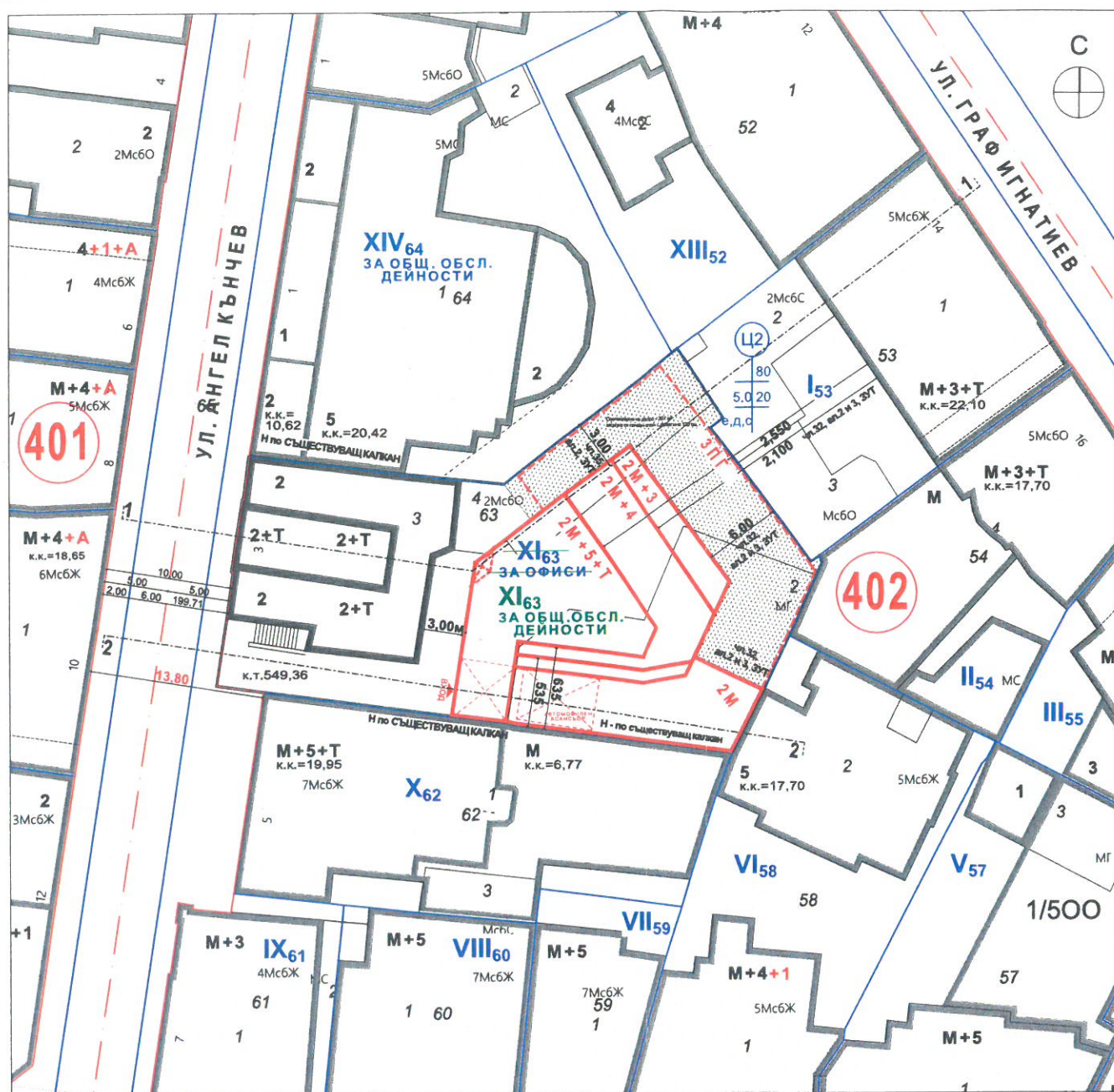
РУП М 1:500
